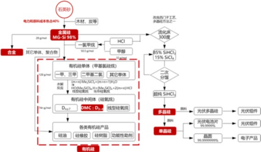
图：含硅材料产业链流程图
